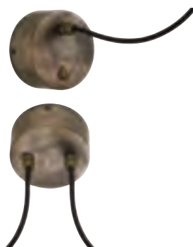
270.06.00 Ø 110 mm H 50 mm Rosone da muro o soffitto con due stringicavo più un tappo. Wall or ceiling canopy with two cable glands and screw top. IP 44
